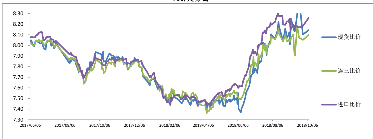
比价走势图
