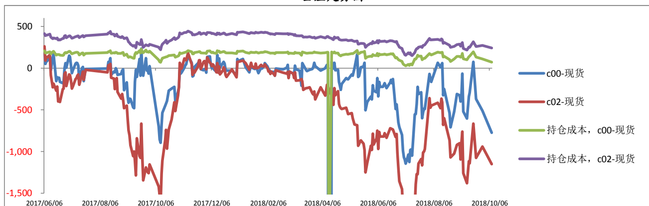
基差走势图
