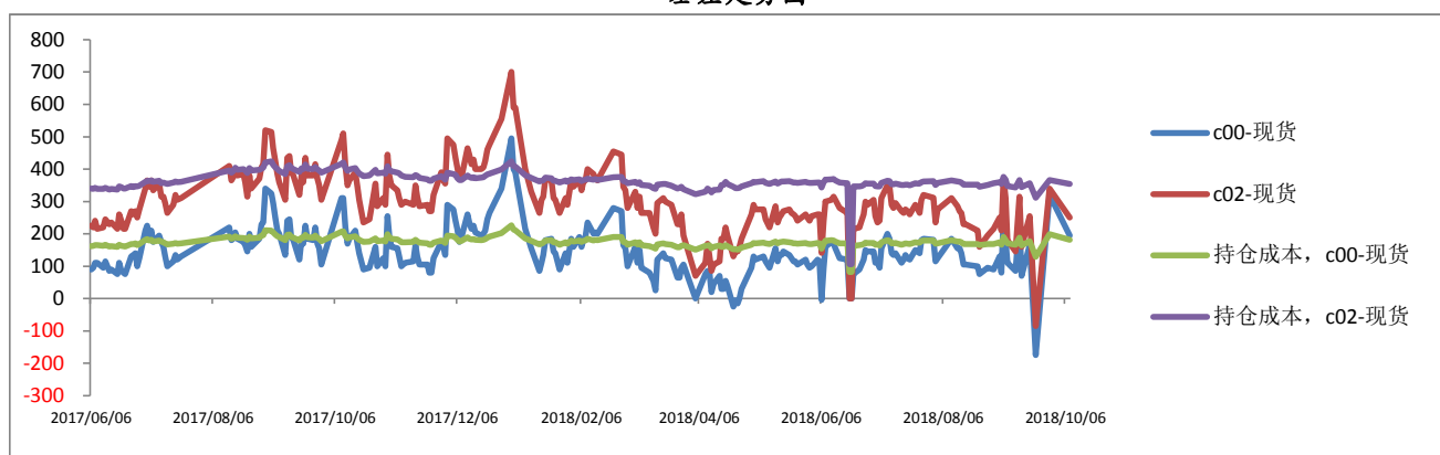
基差走势图
