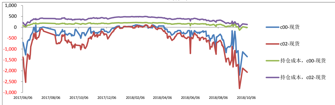
基差走势图
