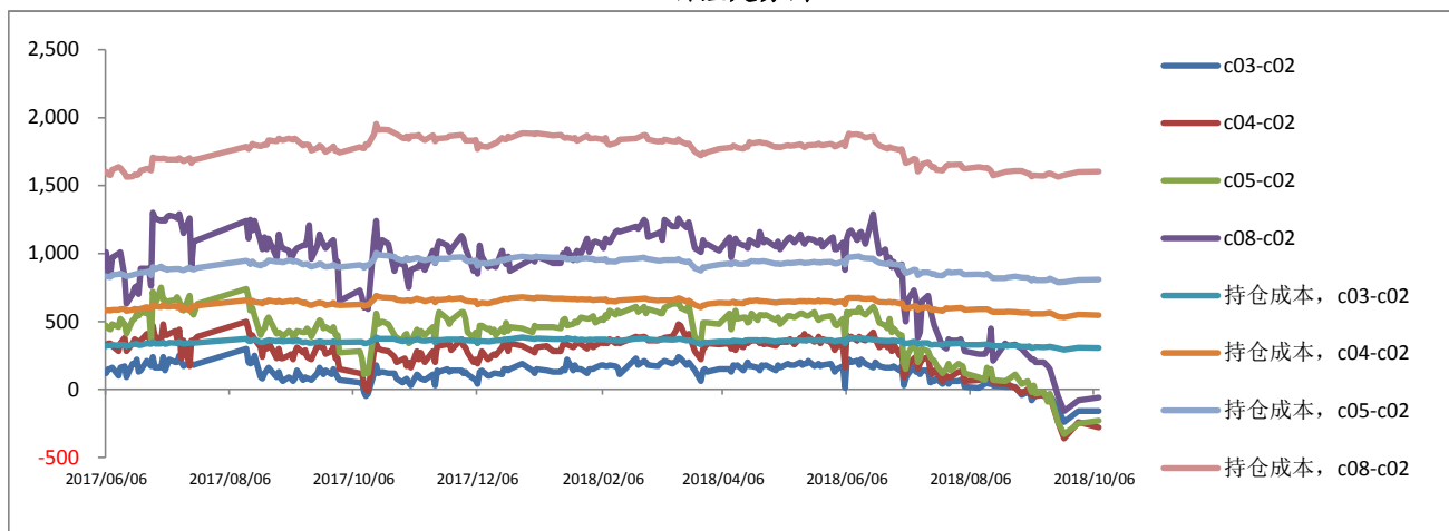
价差走势图
