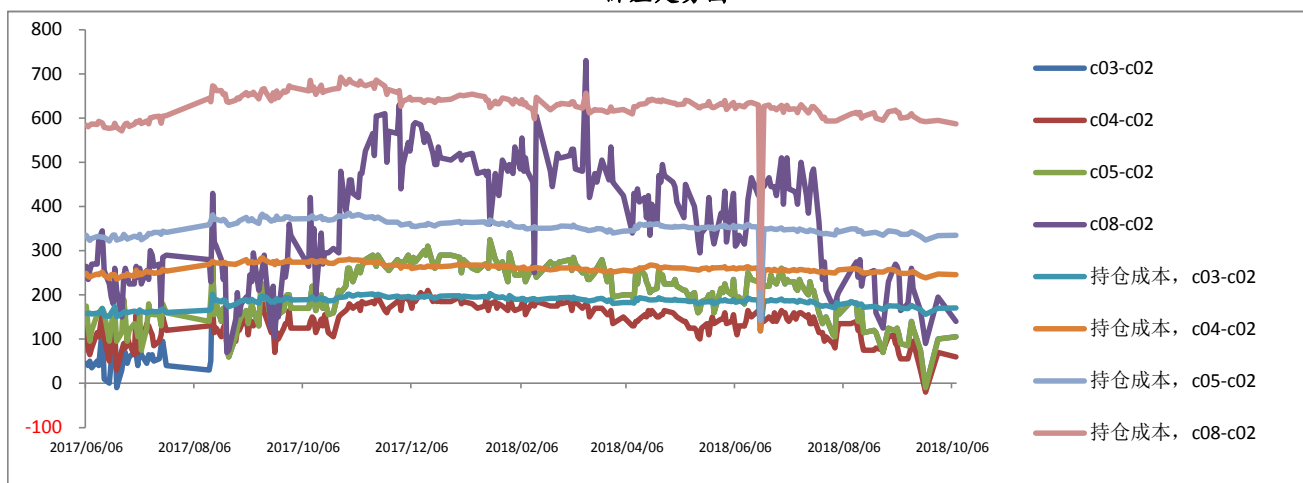
价差走势图
